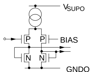
Fig. 4-15: Input pins FBLIN1/2, RIN1/2, BIN1/2, GIN1/2, SENSE
